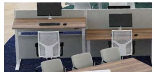
HIRISE 2
